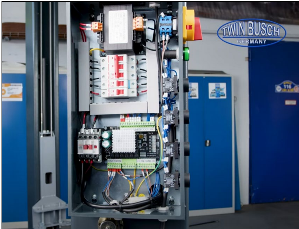
Abbildung: Schaltkasten
