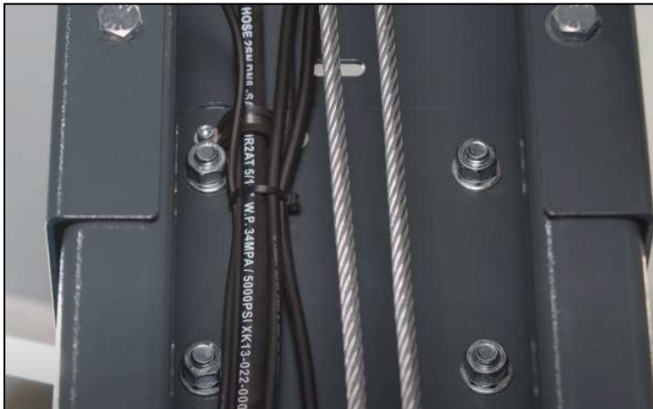
Abbildung: Verlegter Hydraulikschlauch und Kabel
